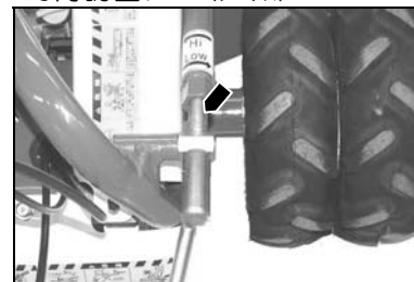
刈高調整レバー(グリス)
