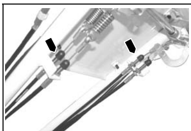
ナイフカバー吊り点(左側)
