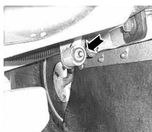
クラッチレバーの支点
