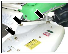
カバー上下リンク支点(左右8箇所)
