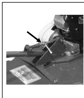
刈高調整ボルト
