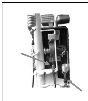
スロットル・変速ワイヤ
