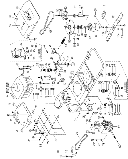
Fig.3 フレーム
