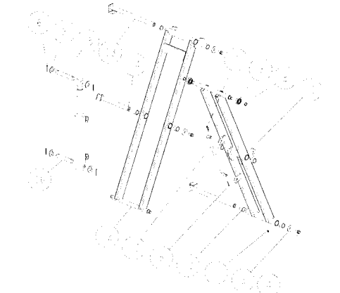
13 Fig.7 リフト部
