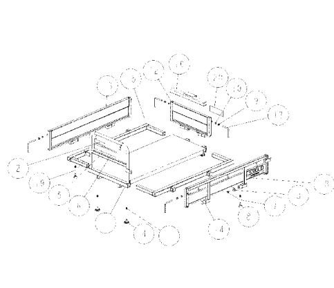
14 Fig.8 荷台部
