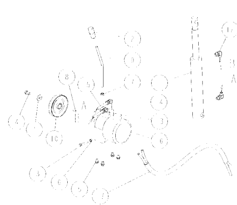
12 Fig.6 油圧部
