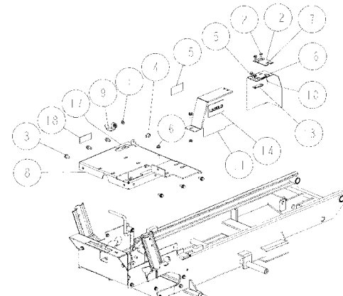
7 Fig.3 フレーム部 1/2
