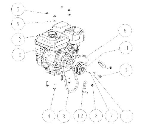
6 Fig.2 エンジン部
