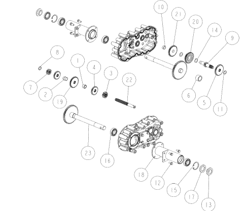
4 Fig.1 ミッション部 4/5
