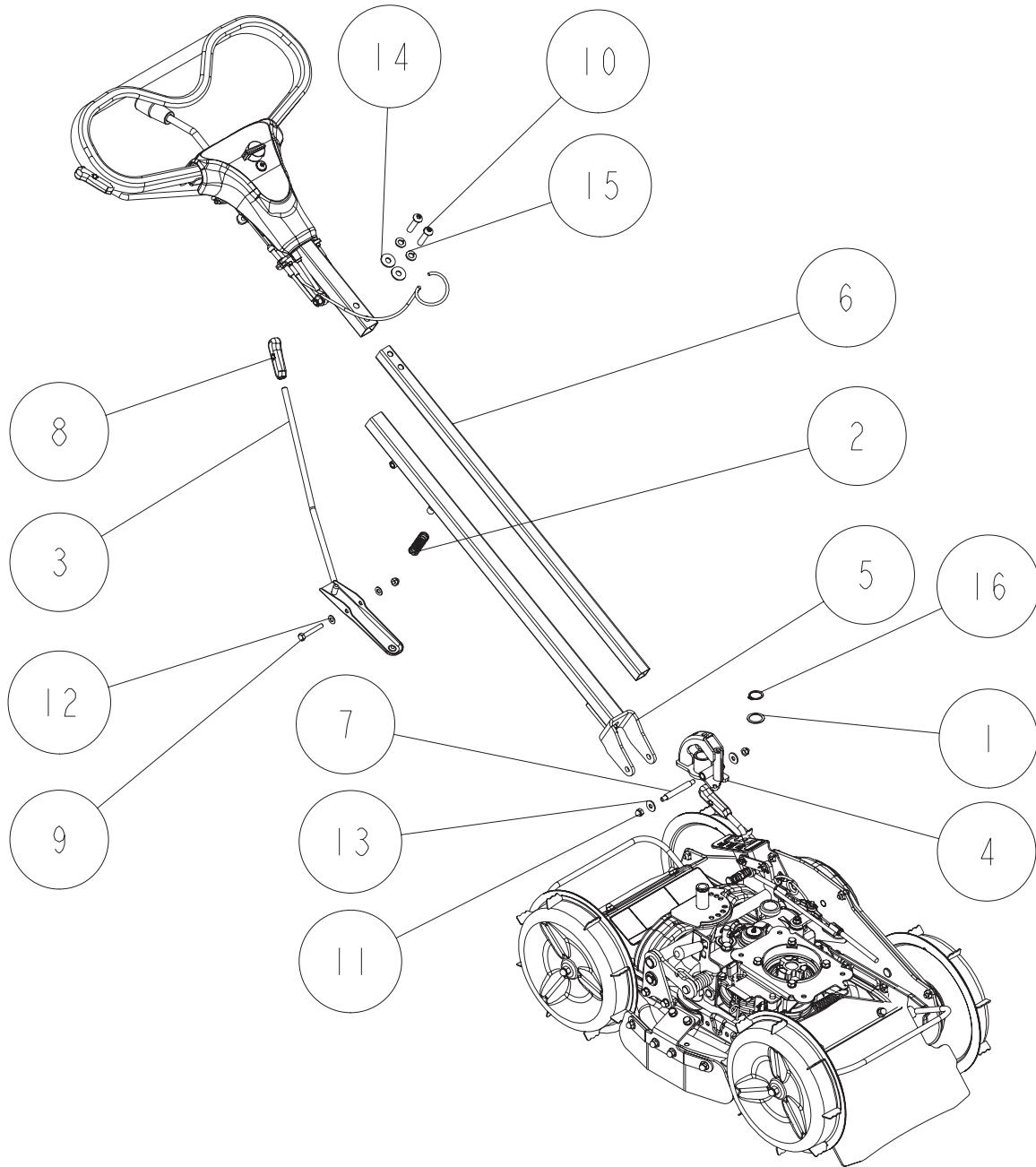
Fig1 ハンドル部-1/3
