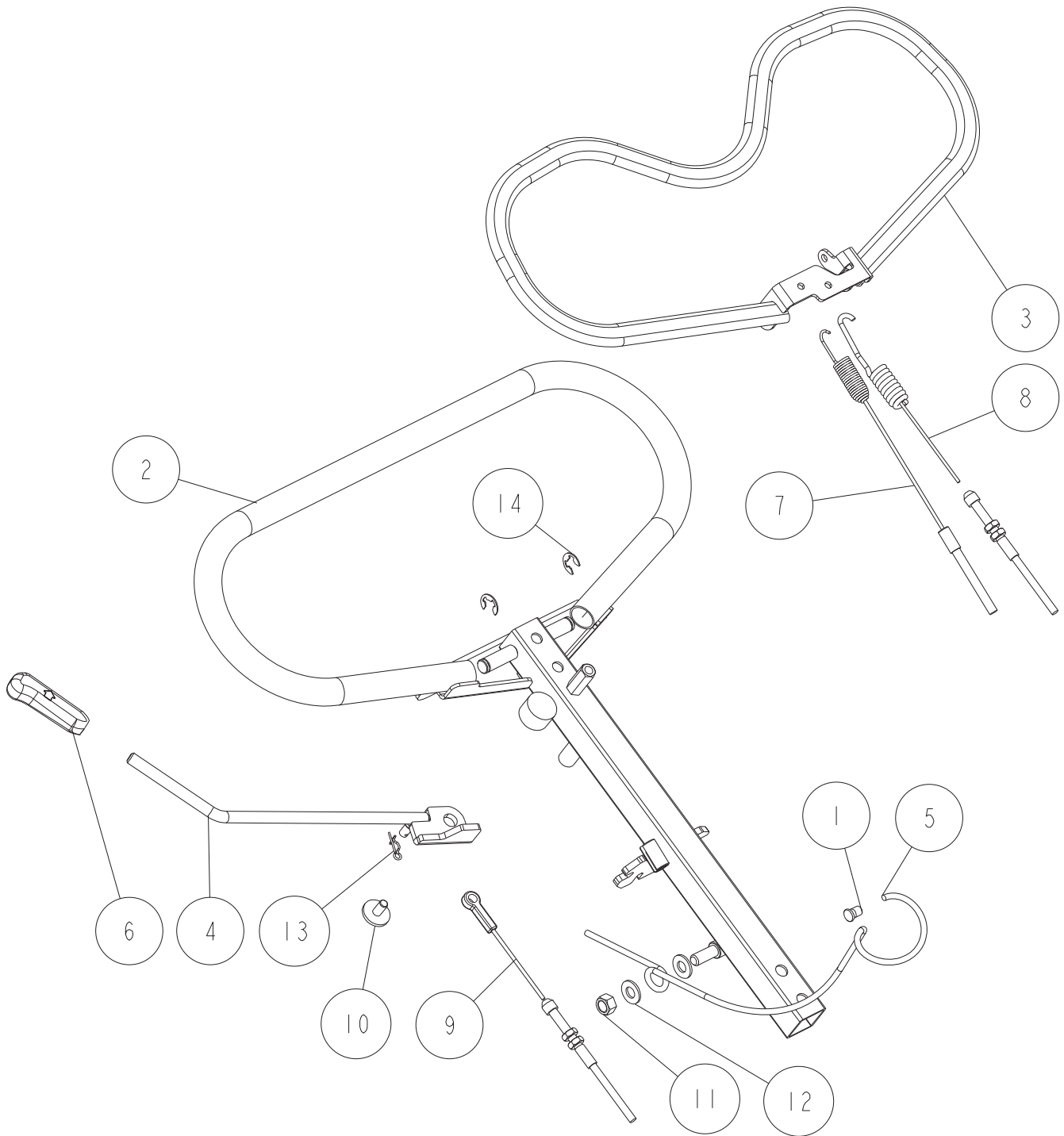
Fig3 ハンドル部-3/3
