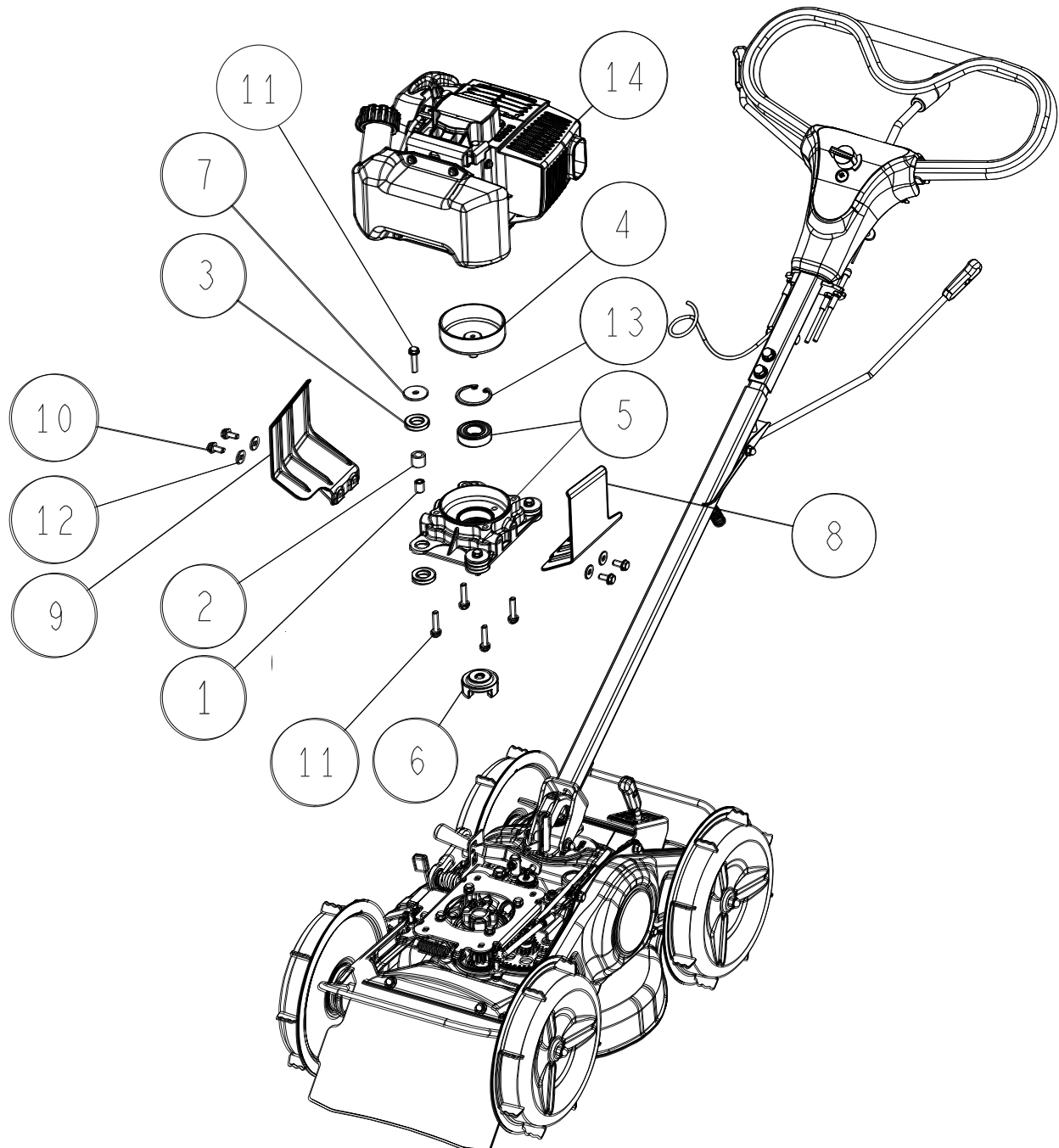
Fig5 エンジン部-1/1
