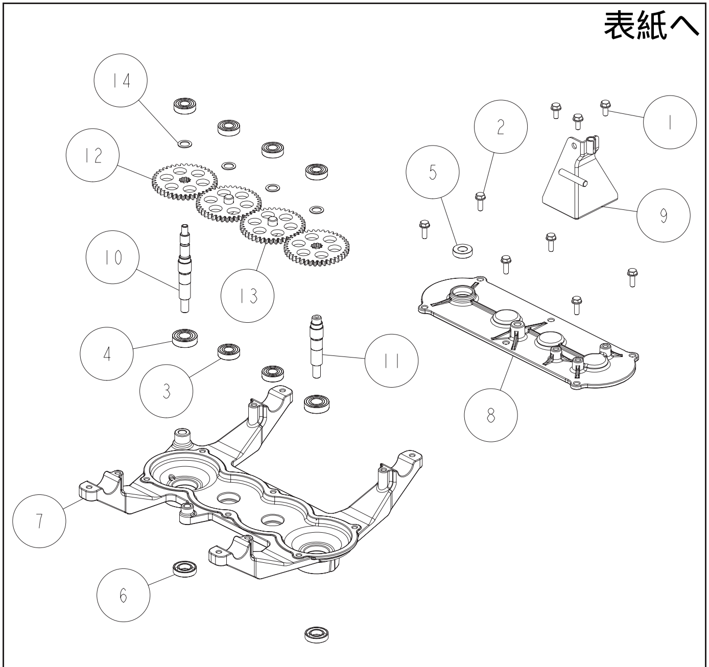
Fig.4-4 刈取部
