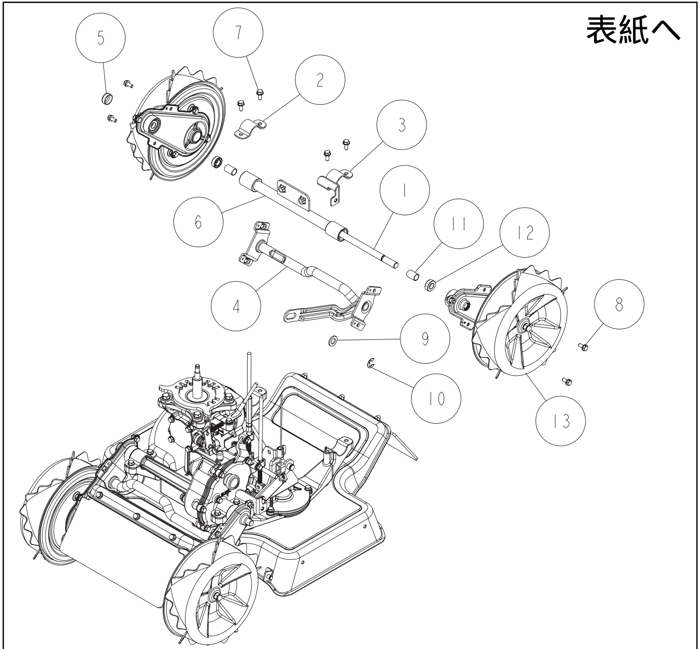
Fig.2-2 駆動部
