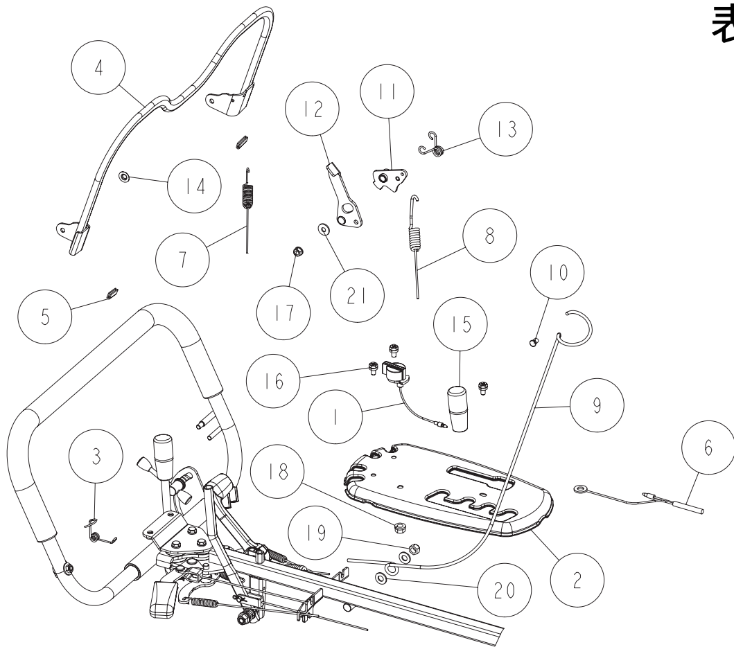
Fig.1-2 ハンドル部
