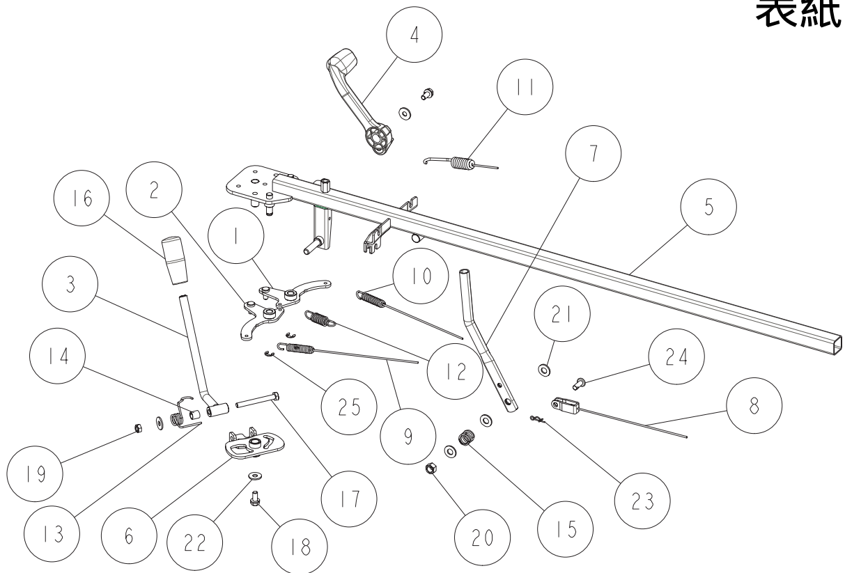
Fig.1-4 ハンドル部
