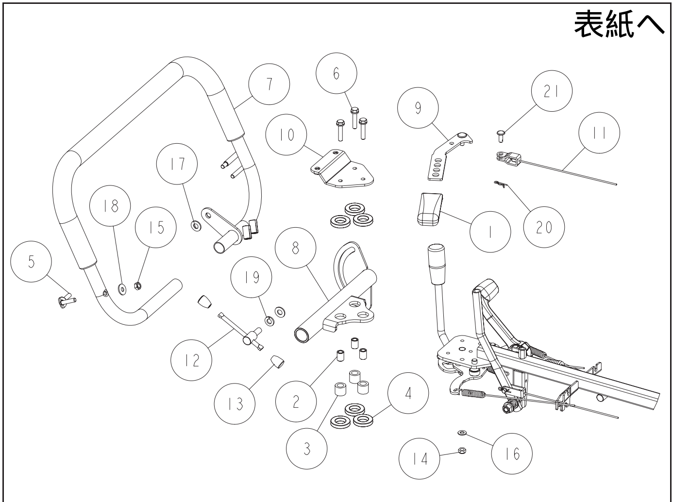
Fig.1-3 ハンドル部
