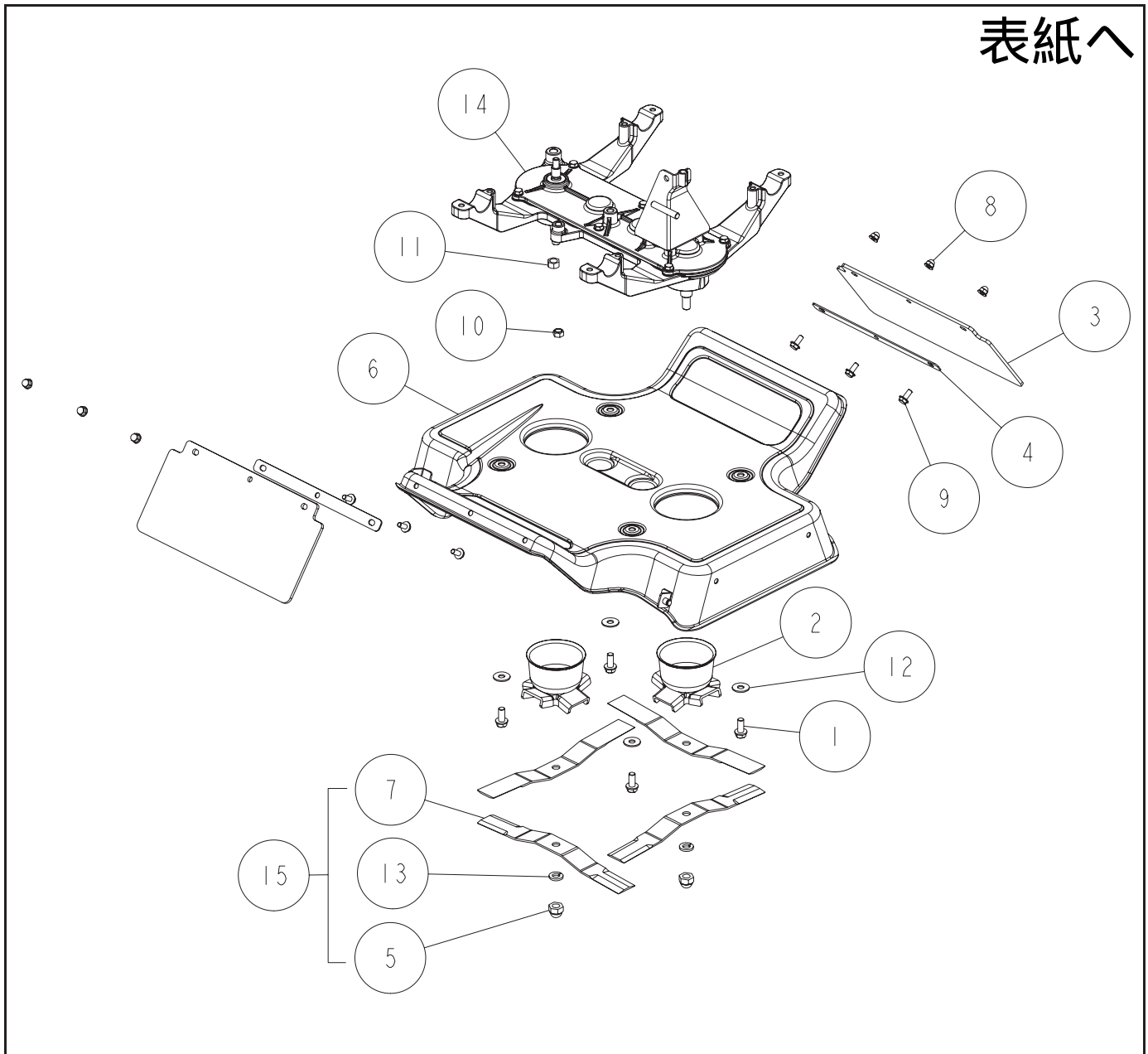
Fig.4-3 刈取部
