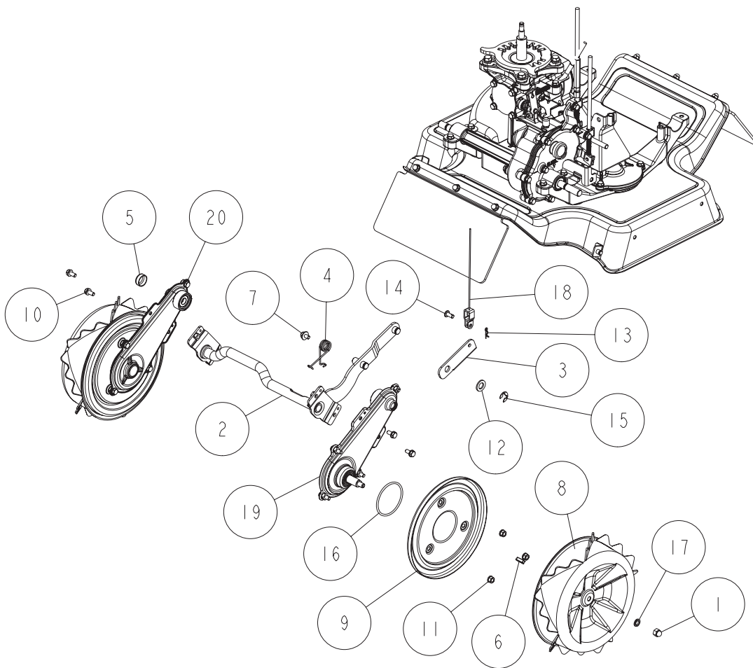
Fig.2-3 駆動部
