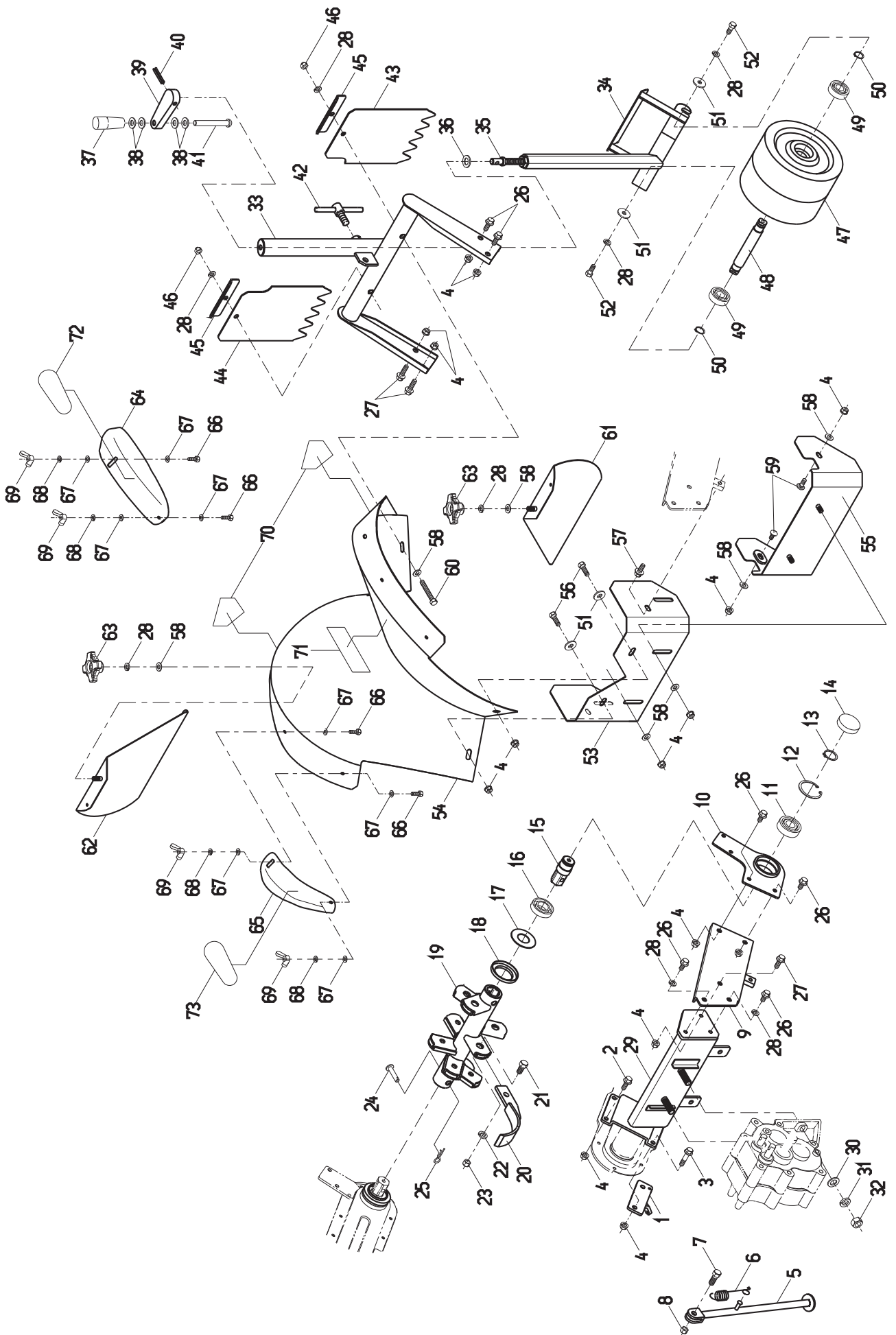
Fig 5 ローター
