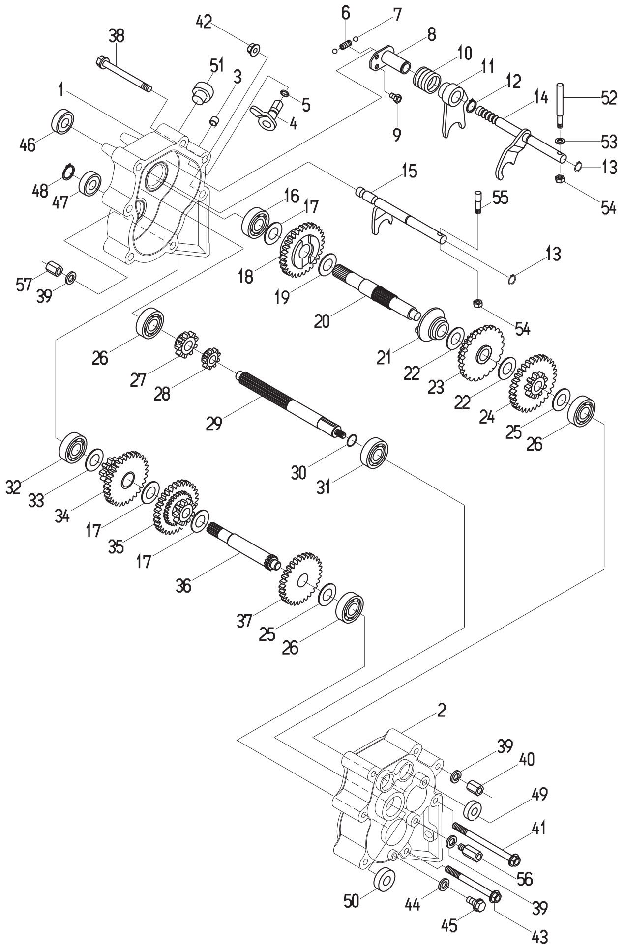
Fig 2 ミッション
