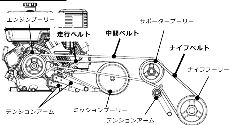
ベルト回り各部名称
