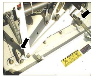
上下リンク支点(左右4ヶ所)
