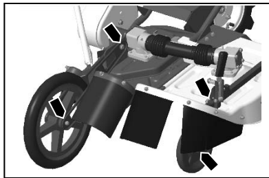
前輪・ガイト車輪支点
