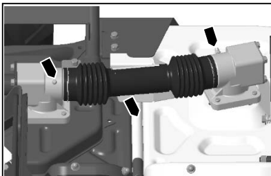
ナイフカバー結合部・ギヤボックス(グリス 40cc)
