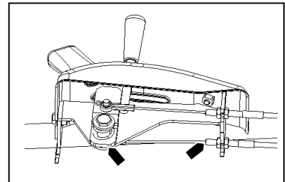
ウイング角度調整ワヤ・レバー支点
