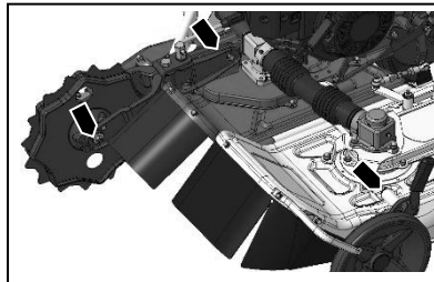
前輪・ガイト車輪支点
