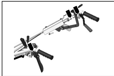
走行・ナイフクラッパヤ・レバー支点
