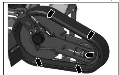
クラ内部・転輪軸(グリス #2)
