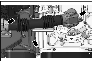
ナイフカバー結合部 ギヤボックス(グリス 30cc)
