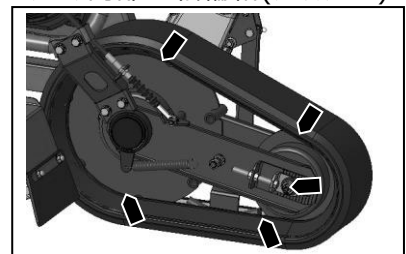
クローラ内部・転輪軸(グリス #2)
