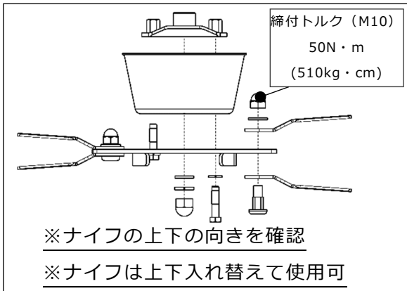
ナイフ分解 側面図
