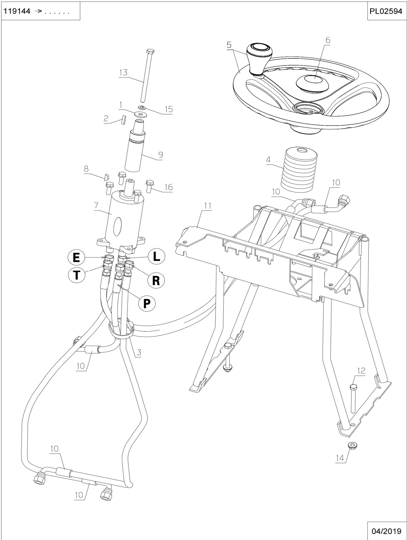
Fig.11-4 ステアリング (機番:EFAJL00004 ~ )
