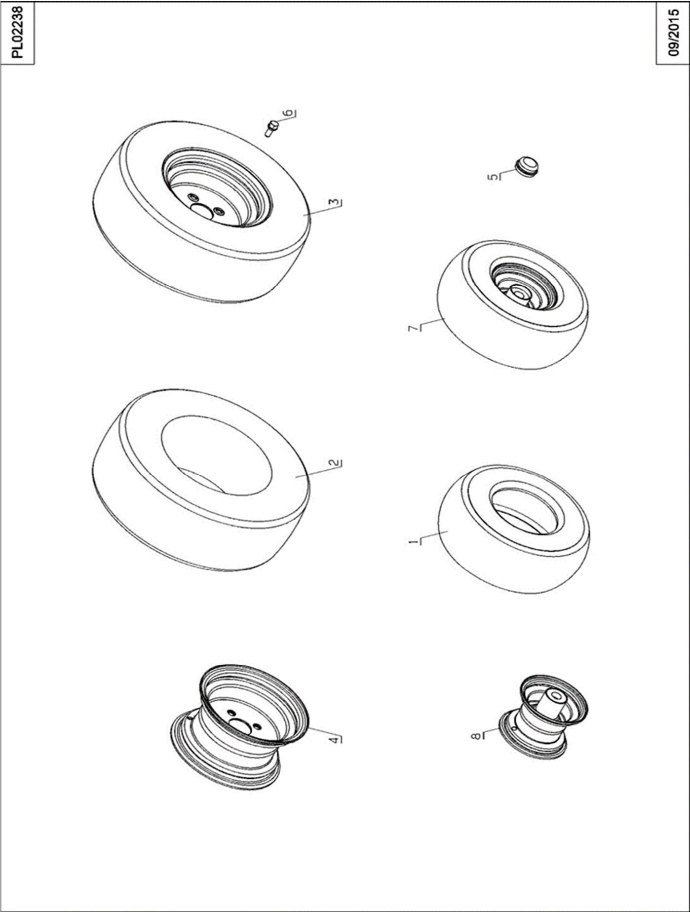
Fig.10 タイヤ
