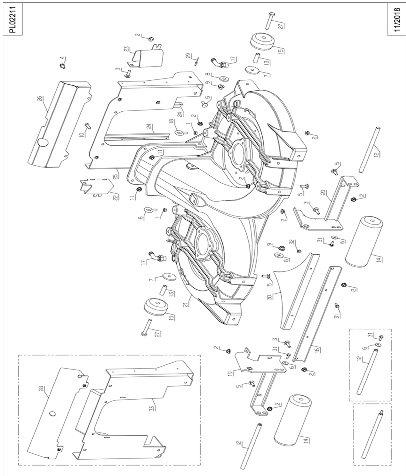
Fig.2 刈取デッキ
