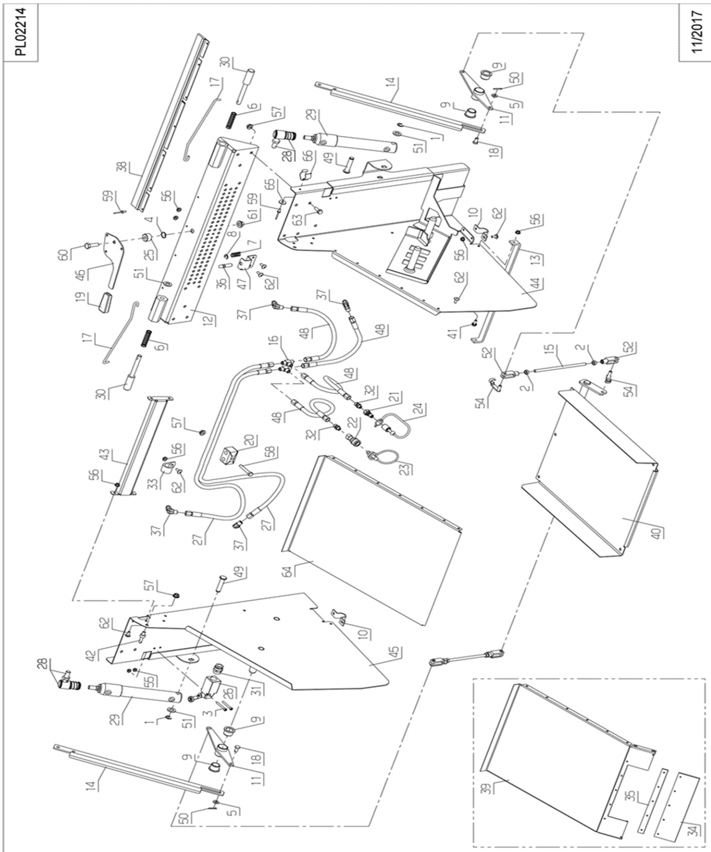
Fig.5 集草ダケ外
