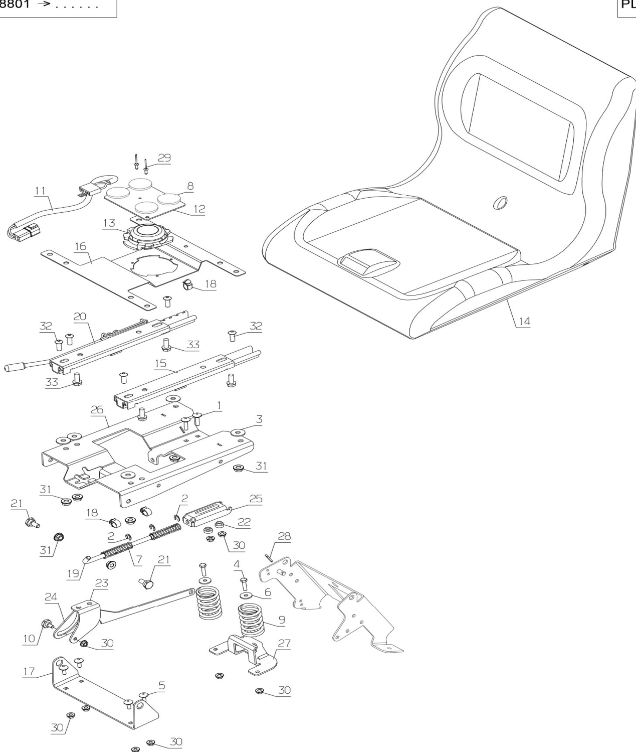
Fig.15-2 シート（機番：EFAJL00004～ ）
