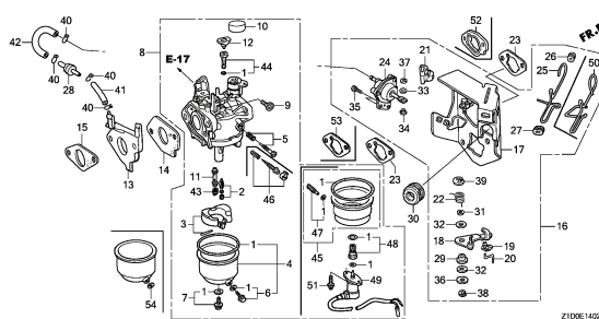
キャブレター (3)
