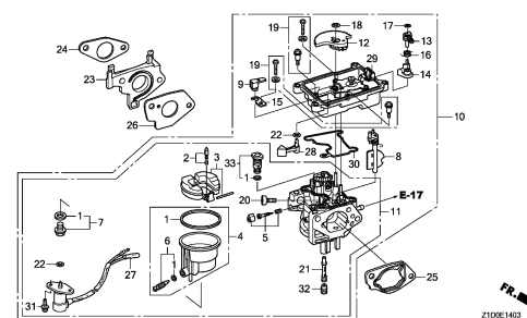
キャブレター (4)
