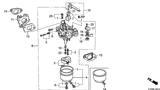
キャブレター (2)
