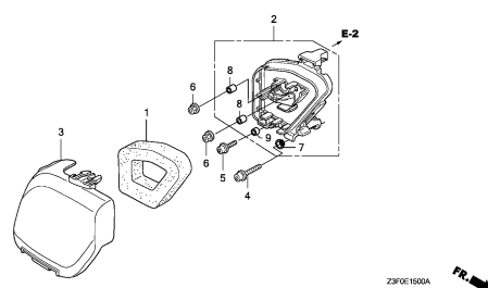
エアークリーナー(1)
