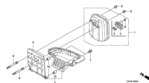
マフラー
