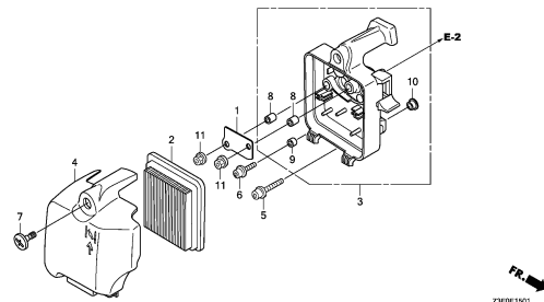
エアークリーナー(2)
