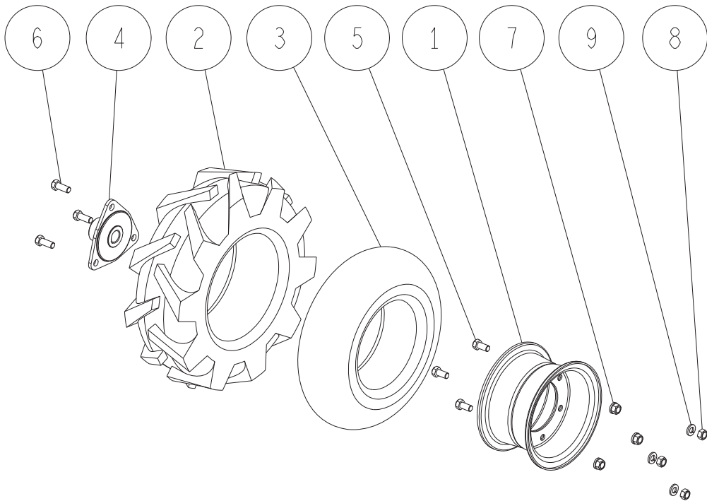
HR400WタイヤセットL
