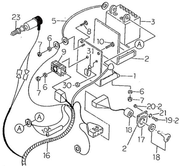
Fig 4 電装品 カワサキ (RM85A)
