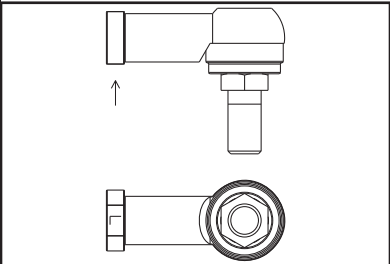
※⑧リンクボール刻印図
