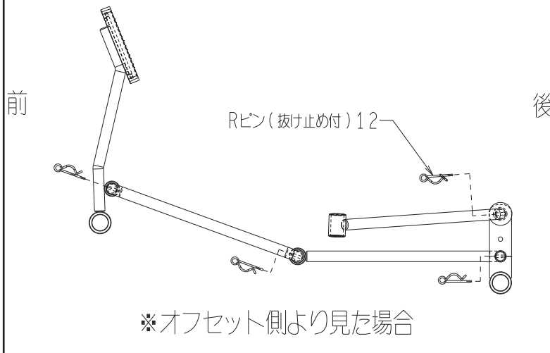
Rピン取付方向図
