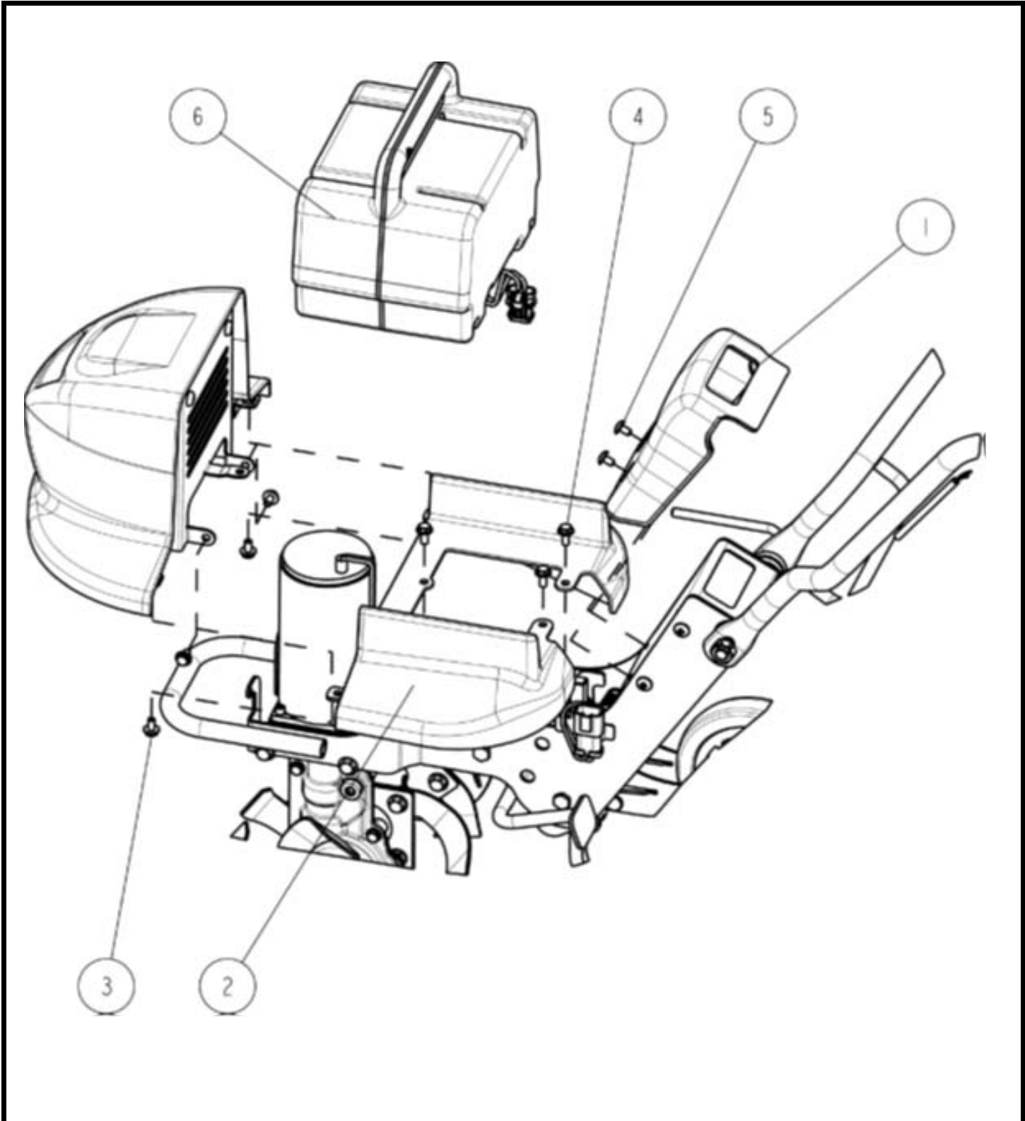
Fig.2 リヤカバー部、バッテリー
