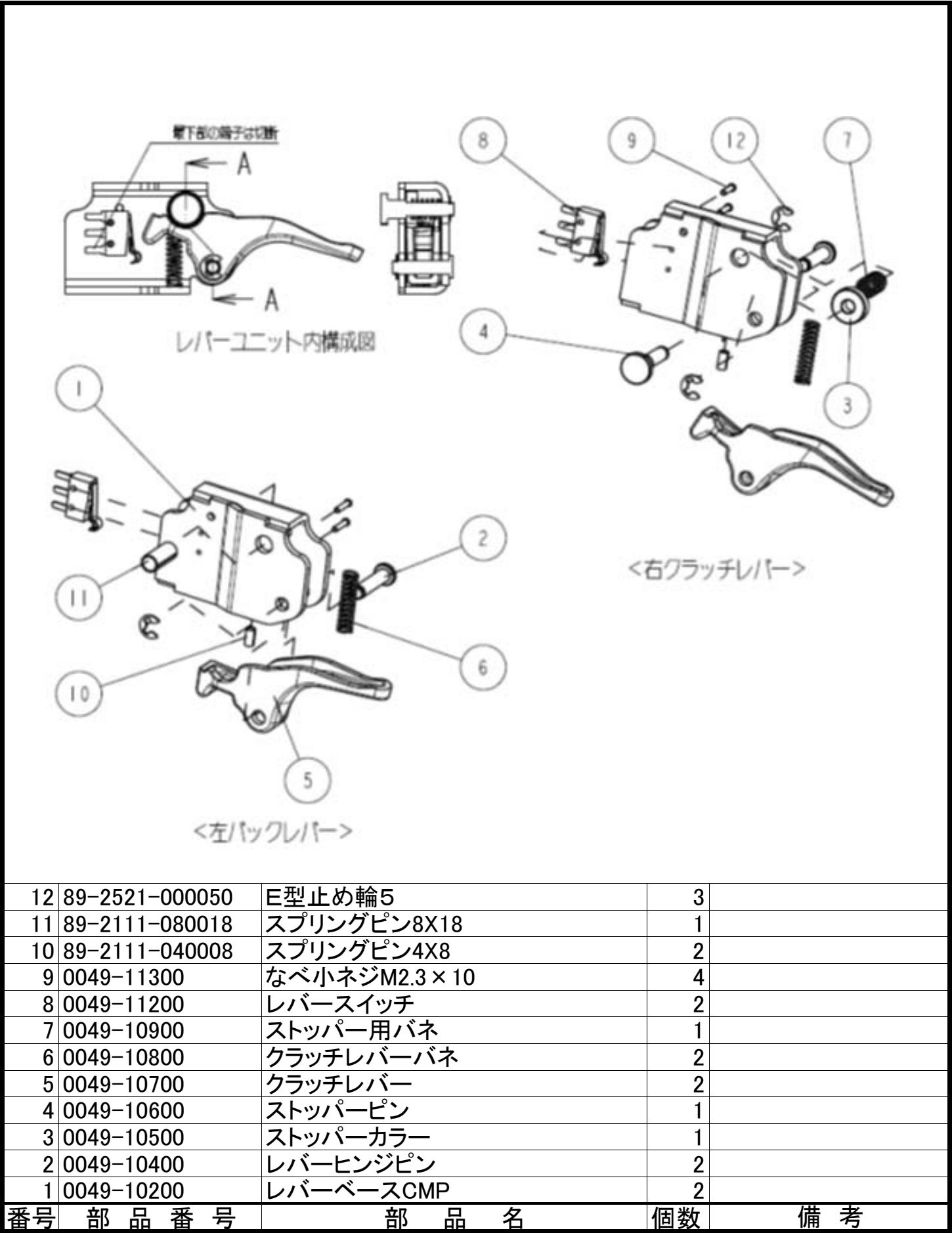
Fig.5 操作レバー部
