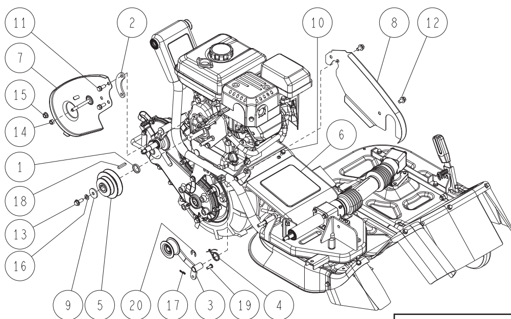
テンションアーム詳細
