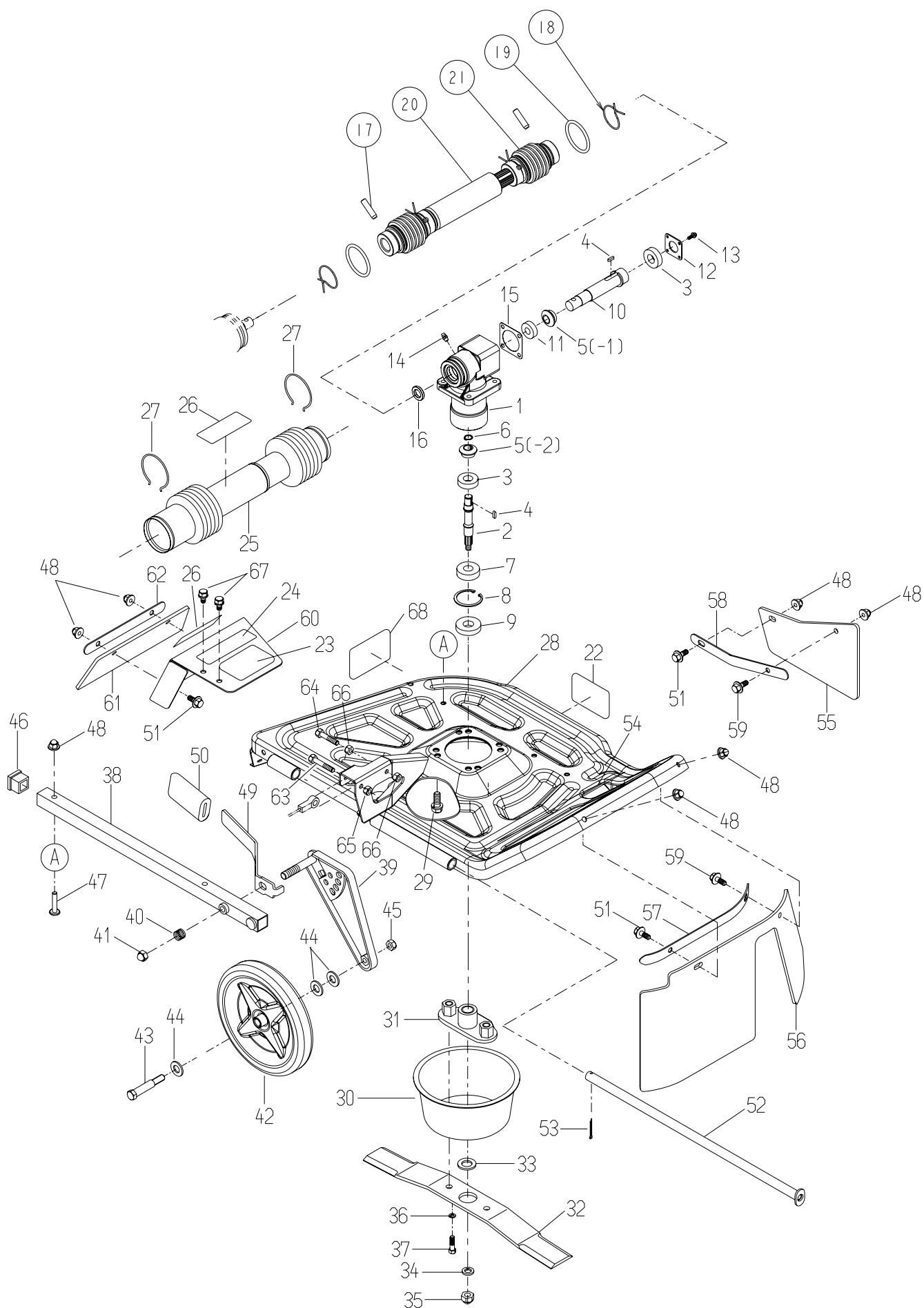
Fig 6 ローターカバー 左
