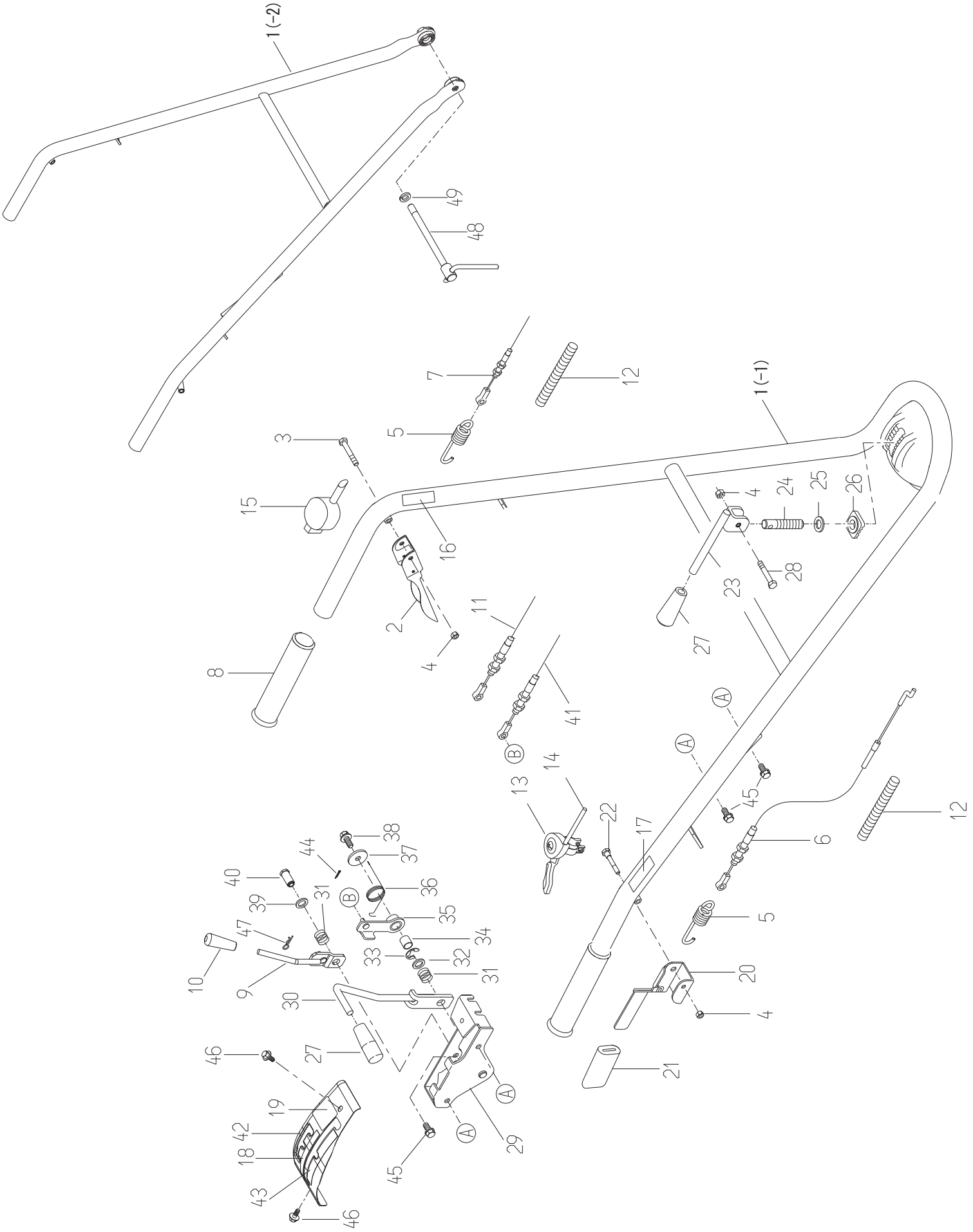
Fig 1 ハンドル
