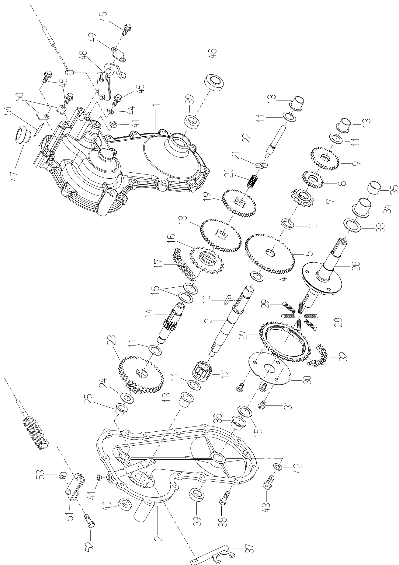
Fig 2 ミッション
