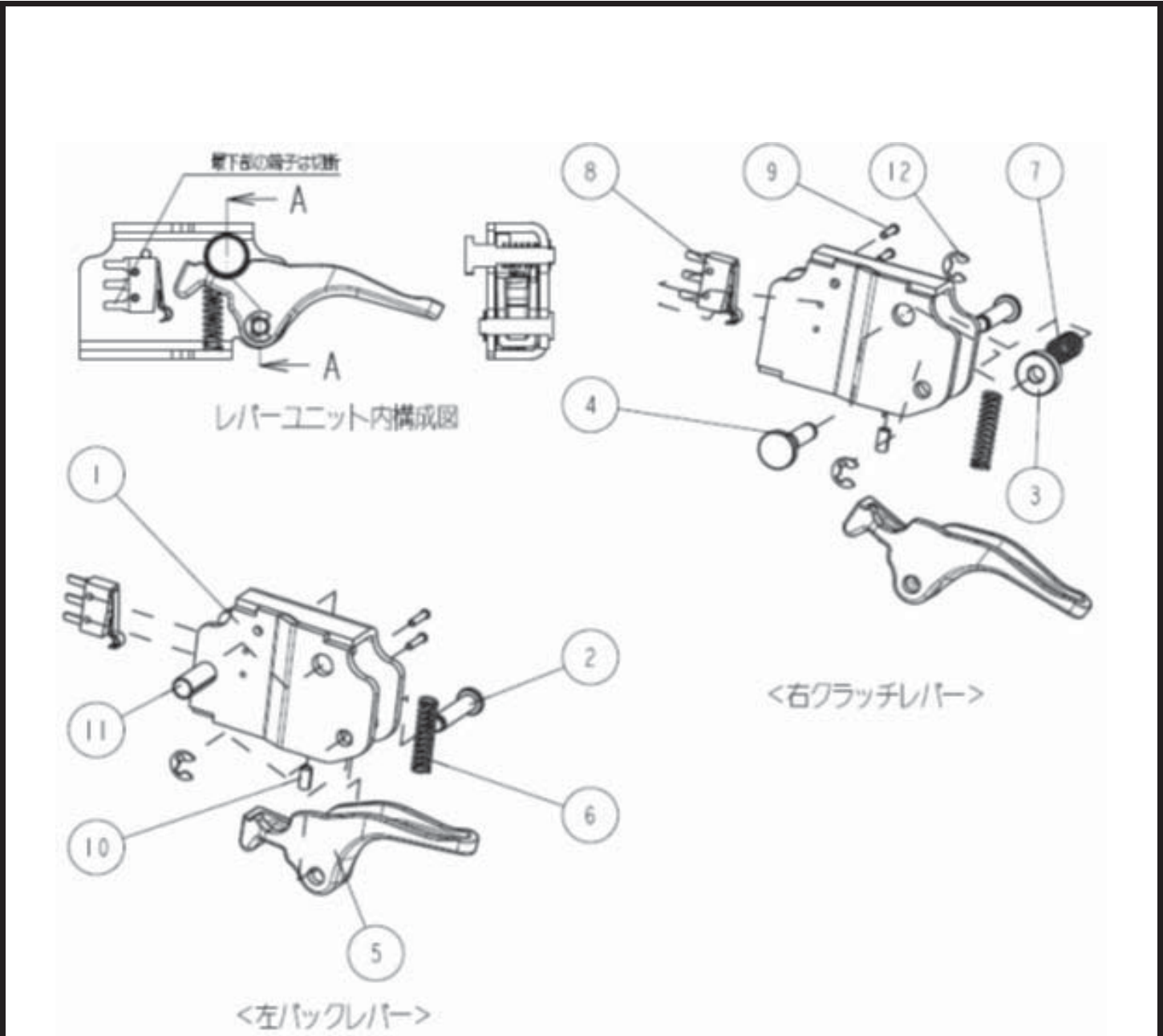
Fig.5 操作レバー部
