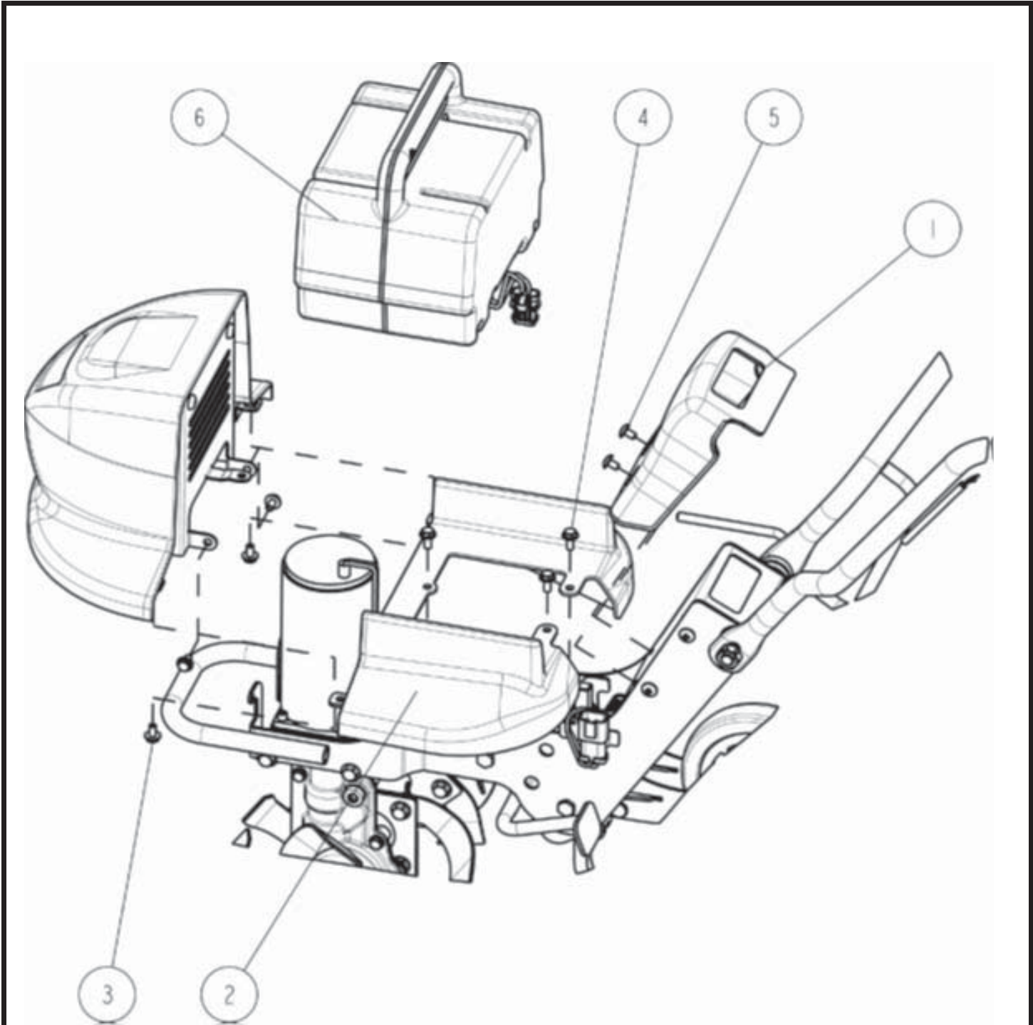
Fig.2 リヤカバー部、バッテリー
