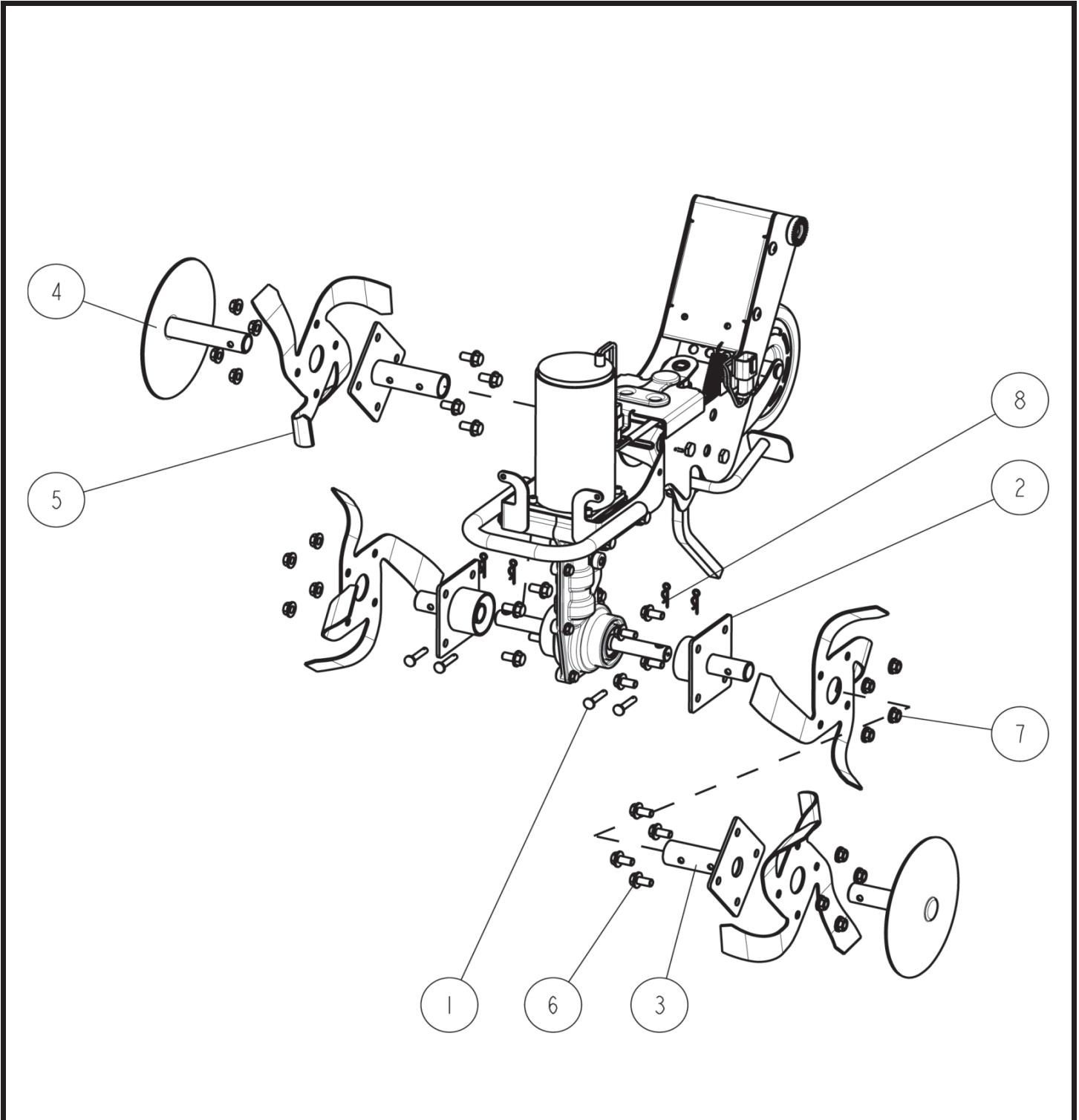
Fig.6 ロータリ一部
